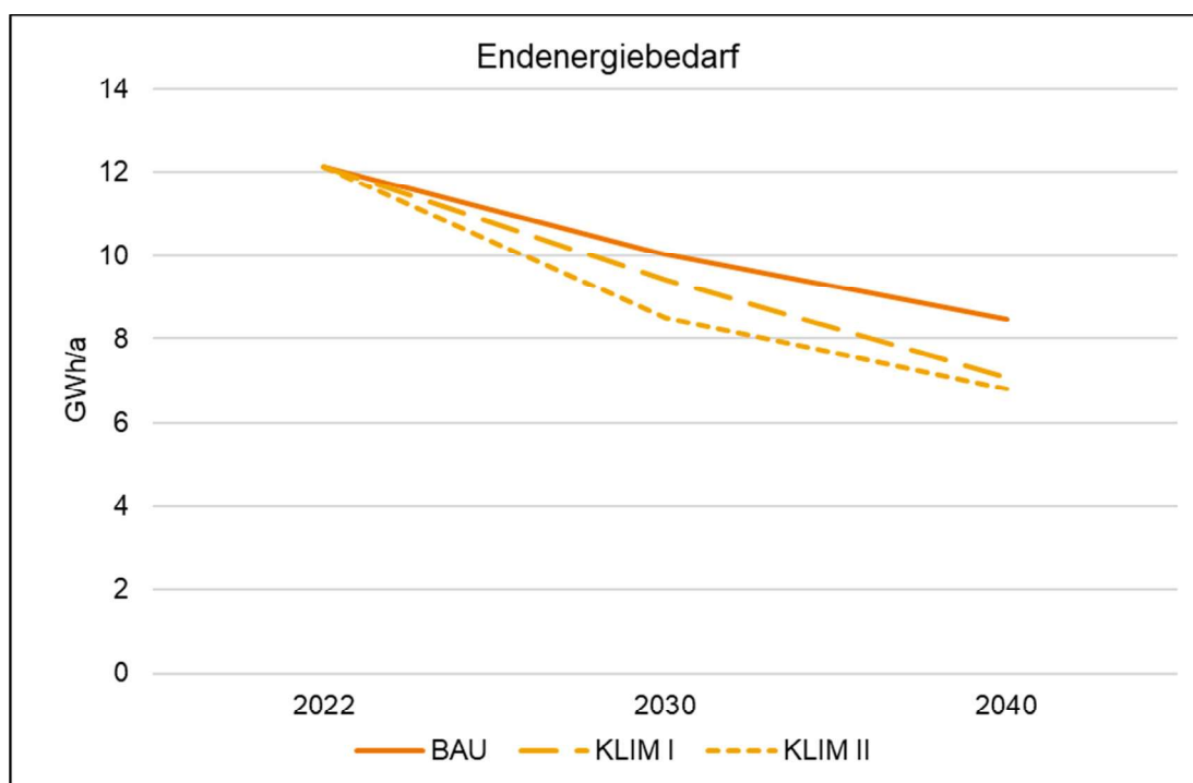
Abbildung 39: Entwicklung des Endenergiebedarfs in den berechneten Szenarien
