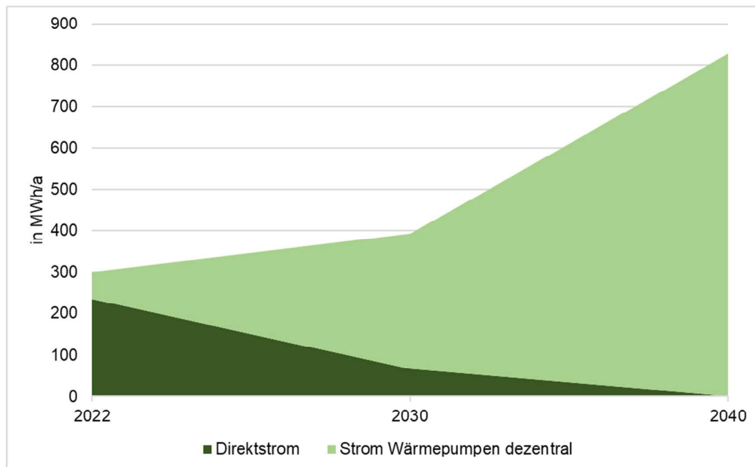
Abbildung 45: Zunahme des Strombedarfs durch Wärmeerzeuger im Zielszenario
