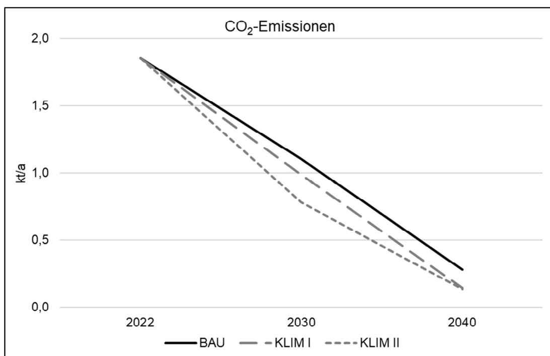
Abbildung 40: Entwicklung der CO 2 -Emissionen in den berechneten Szenarien
