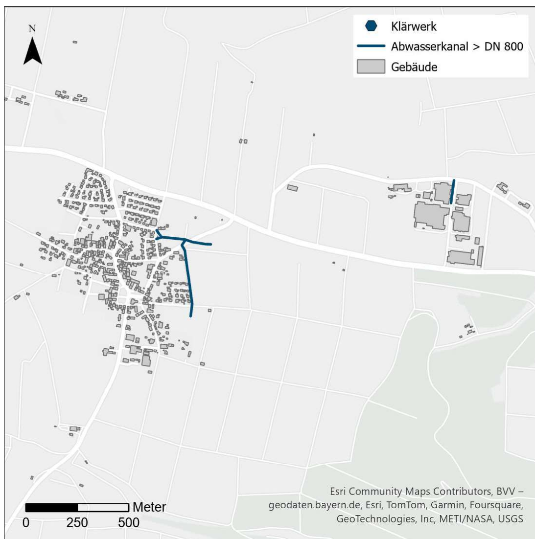
Abbildung 21: Kartografische Darstellung geeigneter Abwassersammler zur Nutzung von Abwasserwärme
