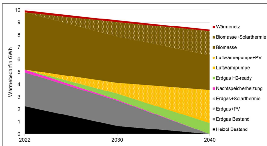
Abbildung 37: Transformation der Wärmebereitstellung im KLIM I-Szenario
