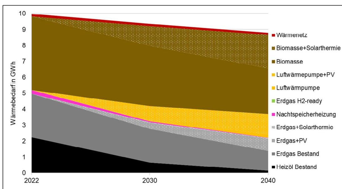
Abbildung 36: Transformation der Wärmebereitstellung im BAU-Szenario
