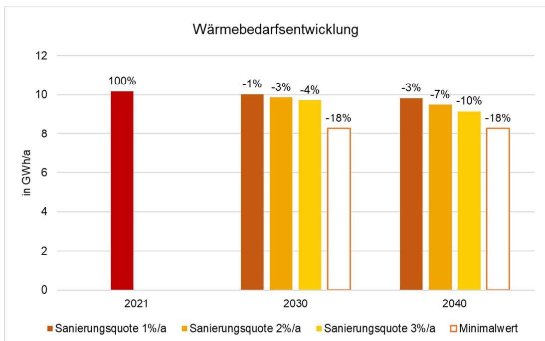
Abbildung 17: Wärmebedarfsreduktion durch Sanierung von Wohngebäuden
