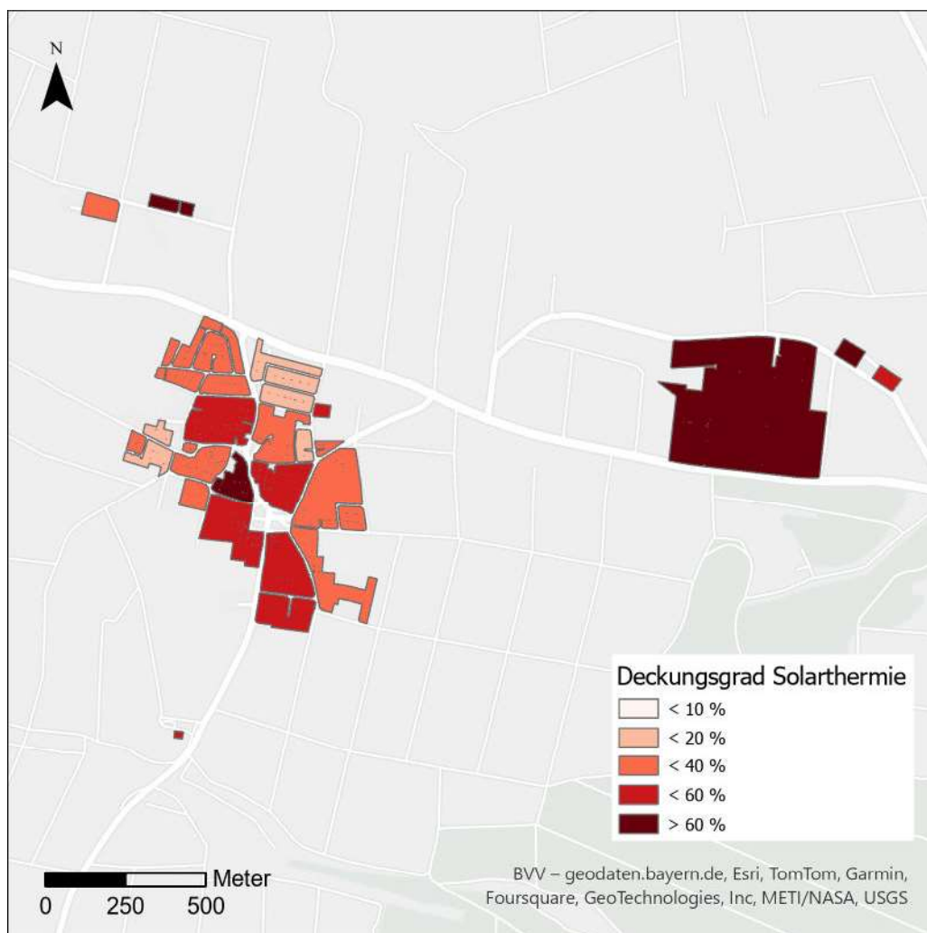
Abbildung 24: Kartografische Darstellung des potenziellen Deckungsgrads von Solarthermie-Anlagen
