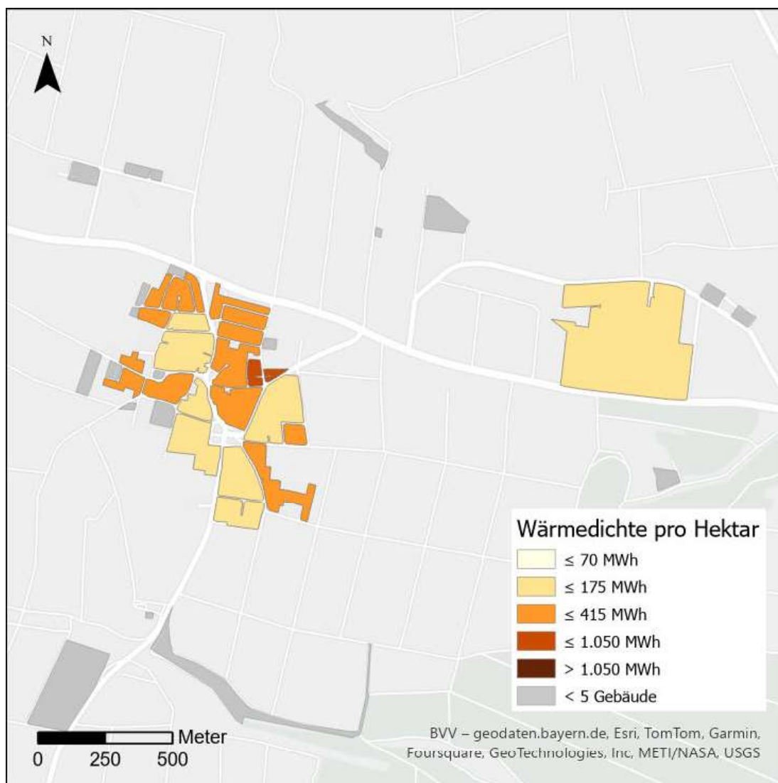
Abbildung 19: Kartografische Darstellung der Wärmedichten im Basisjahr
