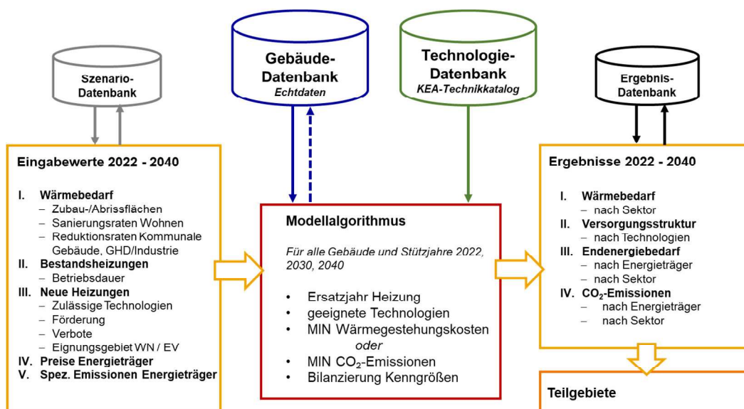
Abbildung 35: Modellstruktur
