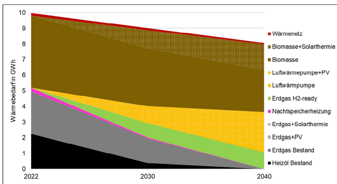
Abbildung 38: Transformation der Wärmebereitstellung im KLIM II-Szenario
